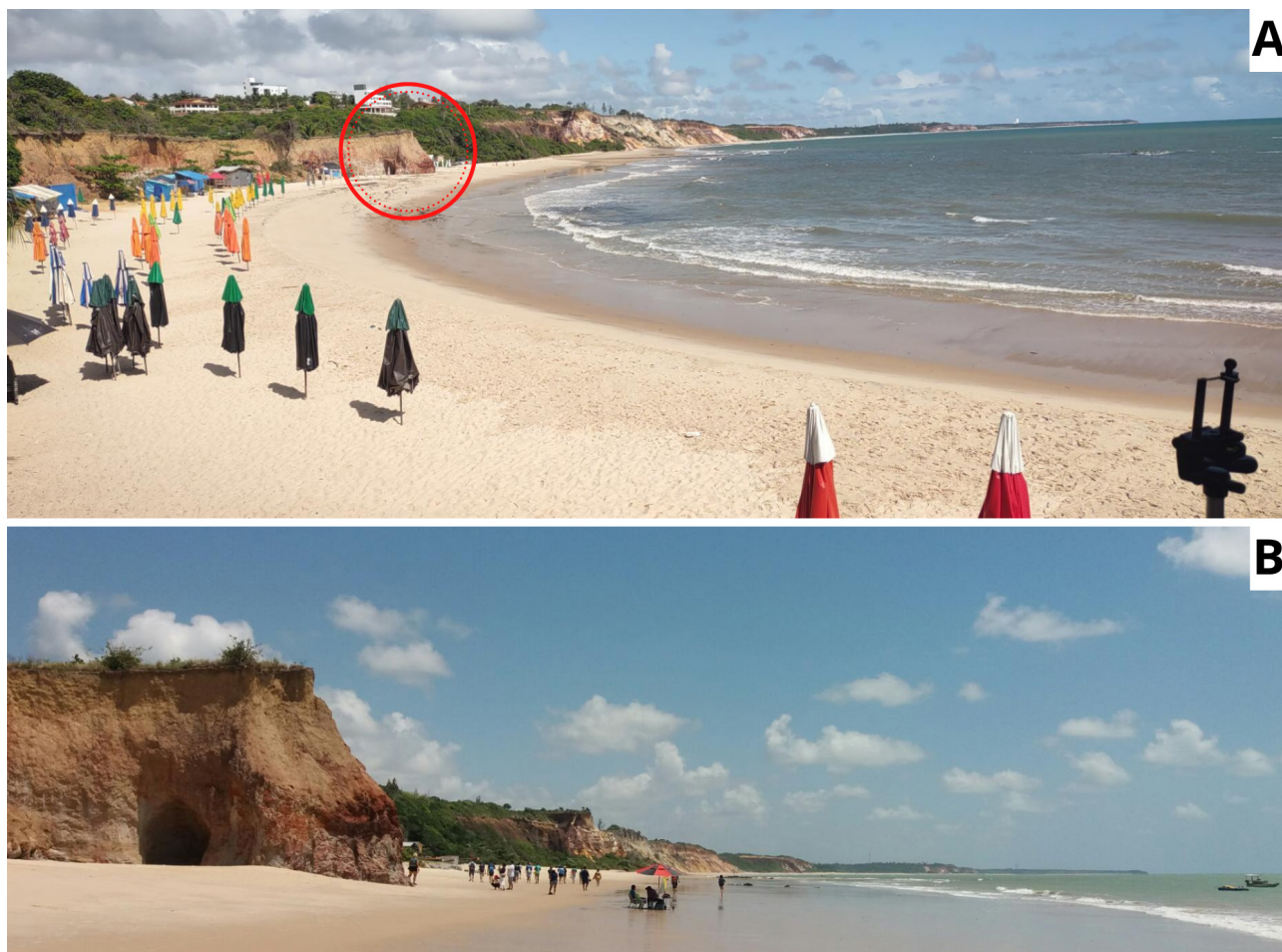
FIGURA 3: Praia do amor em 2022, destaque para abertura da cavidade na ponta da falésia. A) Foto tirada pelo app CoastSnap durante uma ação de monitoramento. B) Foto próxima da cavidade, observa-se proximidade com a linha da costa. Autodescrição: foto faixa de areia de praia com sinalização de erosão costeira.
