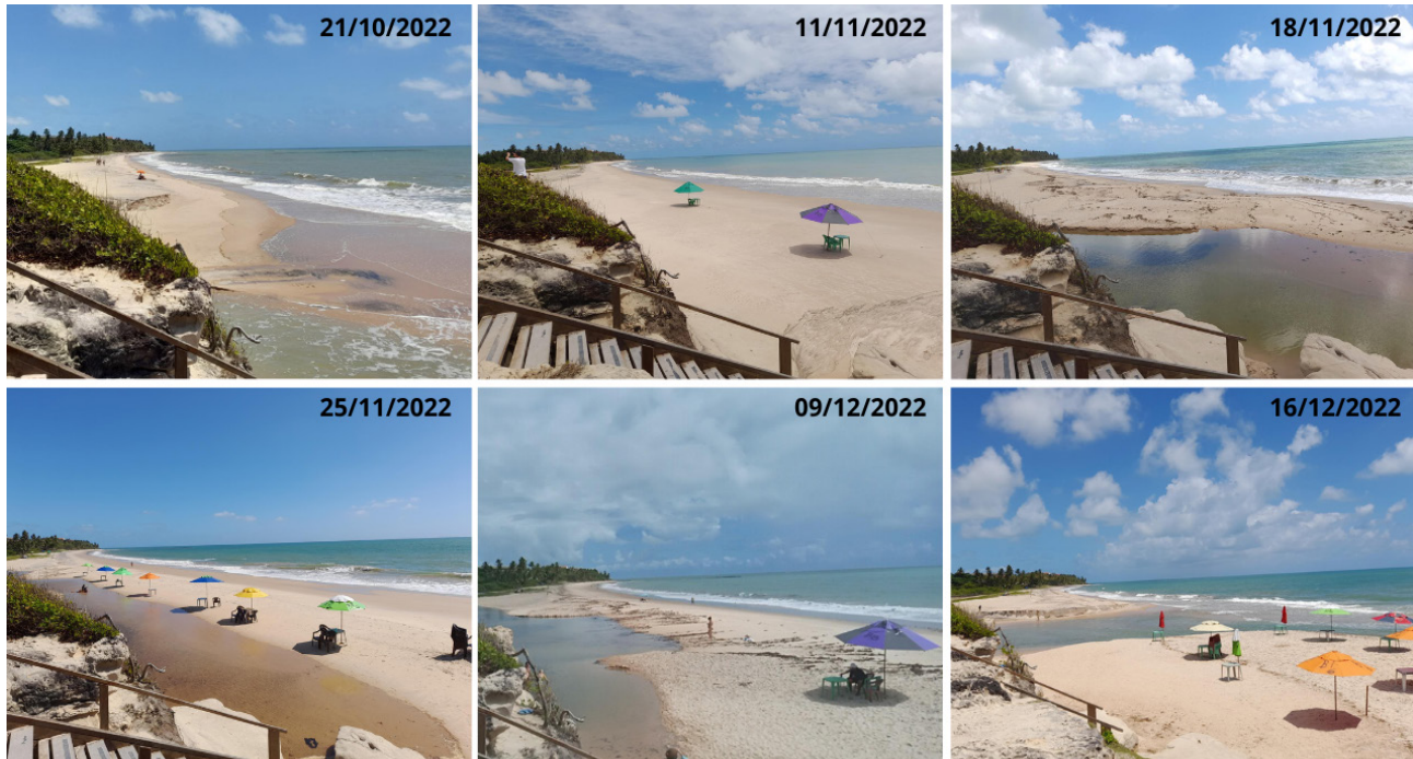
FIGURA 7: Linha do tempo da praia de Tabatinga II face norte. Observam-se as mudanças de direção do canal de maré. Autodescrição: fotos de variação da linha da maré em praia.
